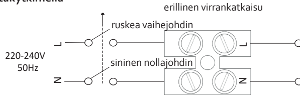
Kuva 1. Kuivain ajastinvirtakytkimellä
